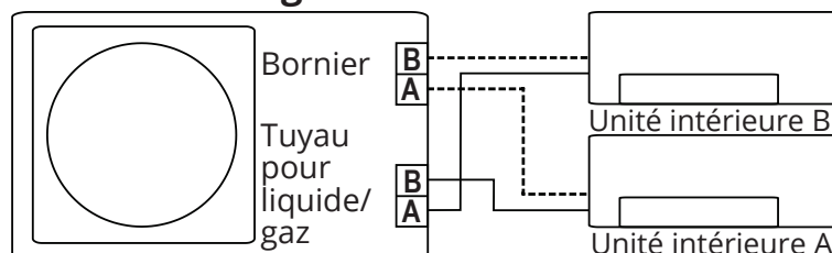
Unité extérieure
